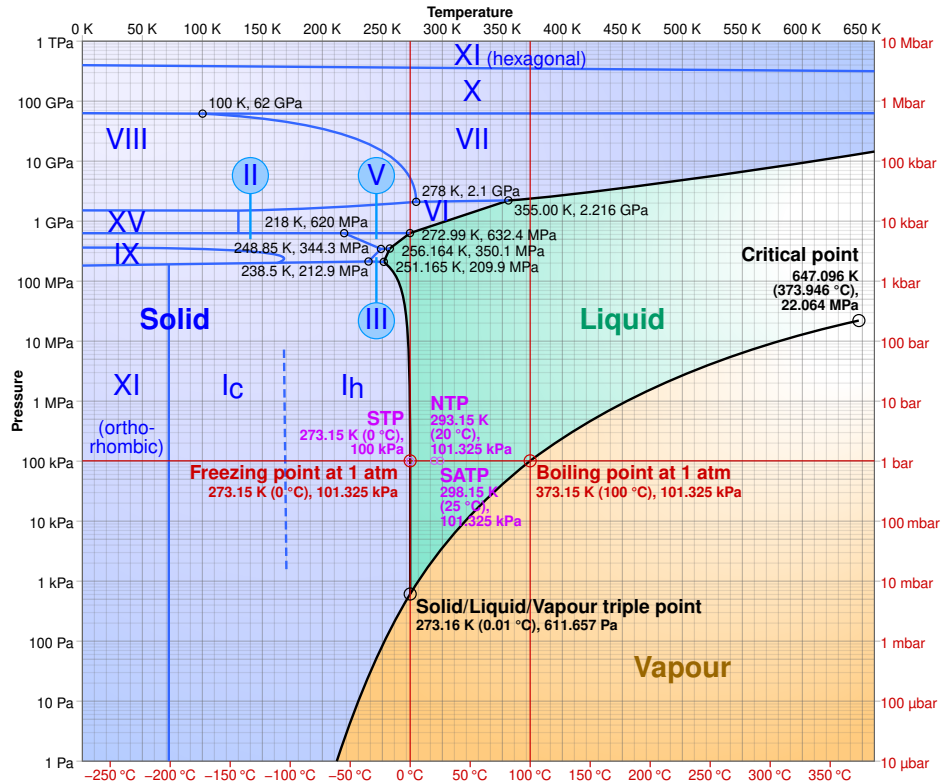
图 12: 冰的相图
