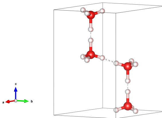
图 13: 冰-I h 的晶体结构 P6_3/mmc a = b = 450.6 \text{ pm}, c = 734.6 \text{ pm}
